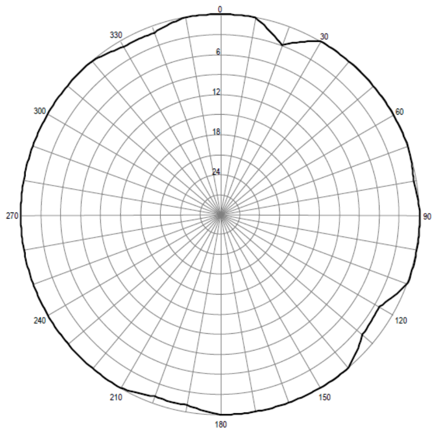
Pozioma charakterystyka promieniowania anteny stacji Sędławki 90,90 MHz
