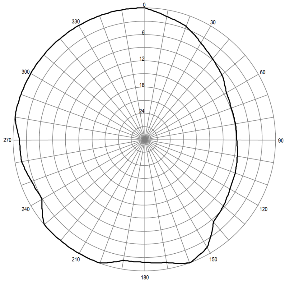
Pozioma charakterystyka promieniowania anteny stacji Poznań 89,80 MHz
