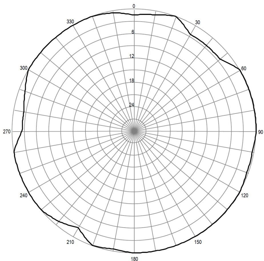
Pozioma charakterystyka promieniowania anteny stacji Leszno 90,20 MHz
