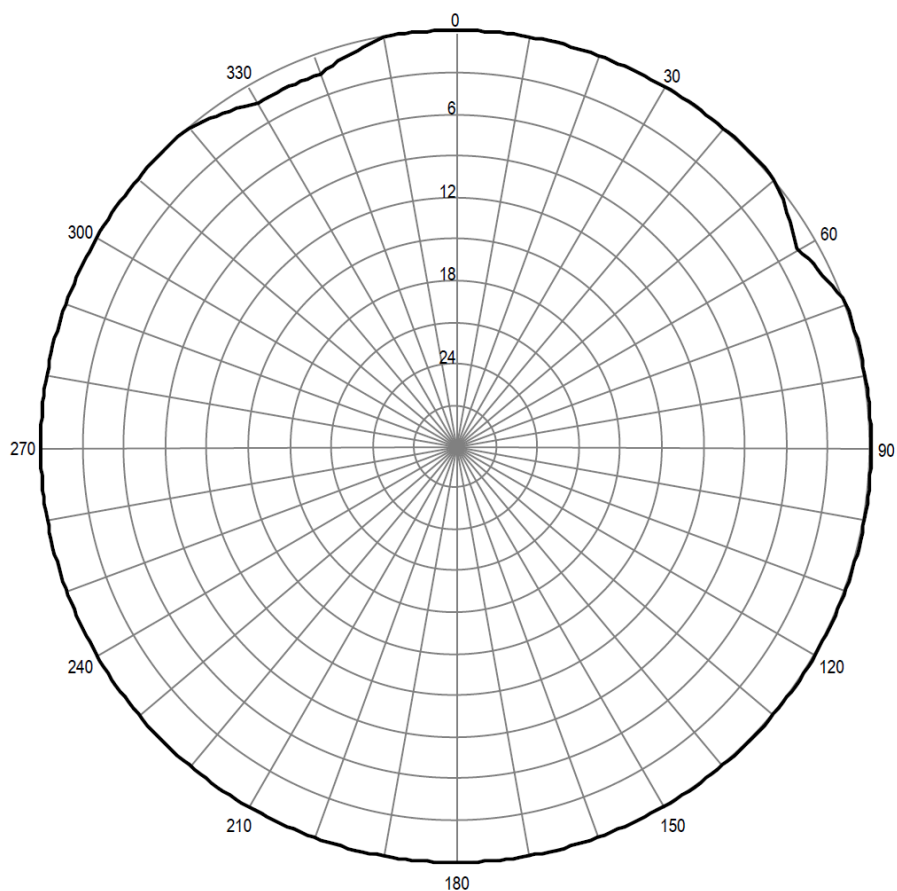
Pozioma charakterystyka promieniowania anteny stacji Olsztyn 88,10 MHz
