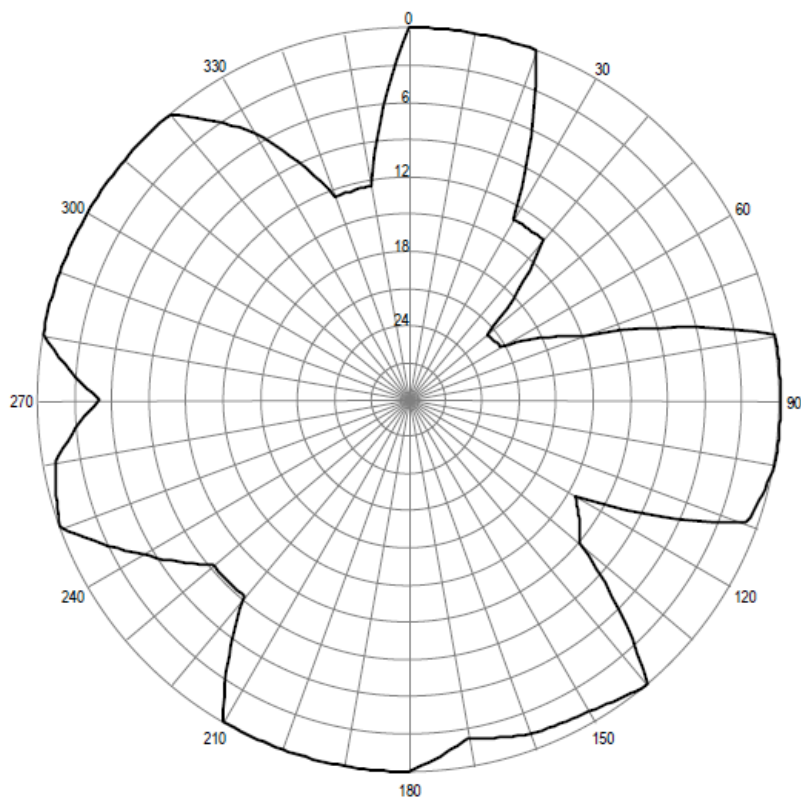
Pozioma charakterystyka promieniowania anteny stacji Bydgoszcz 90,50 MHz
