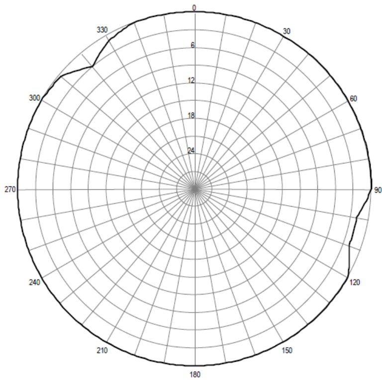
Pozioma charakterystyka promieniowania anteny stacji Kędzierzyn-Koźle 97,70 MHz
