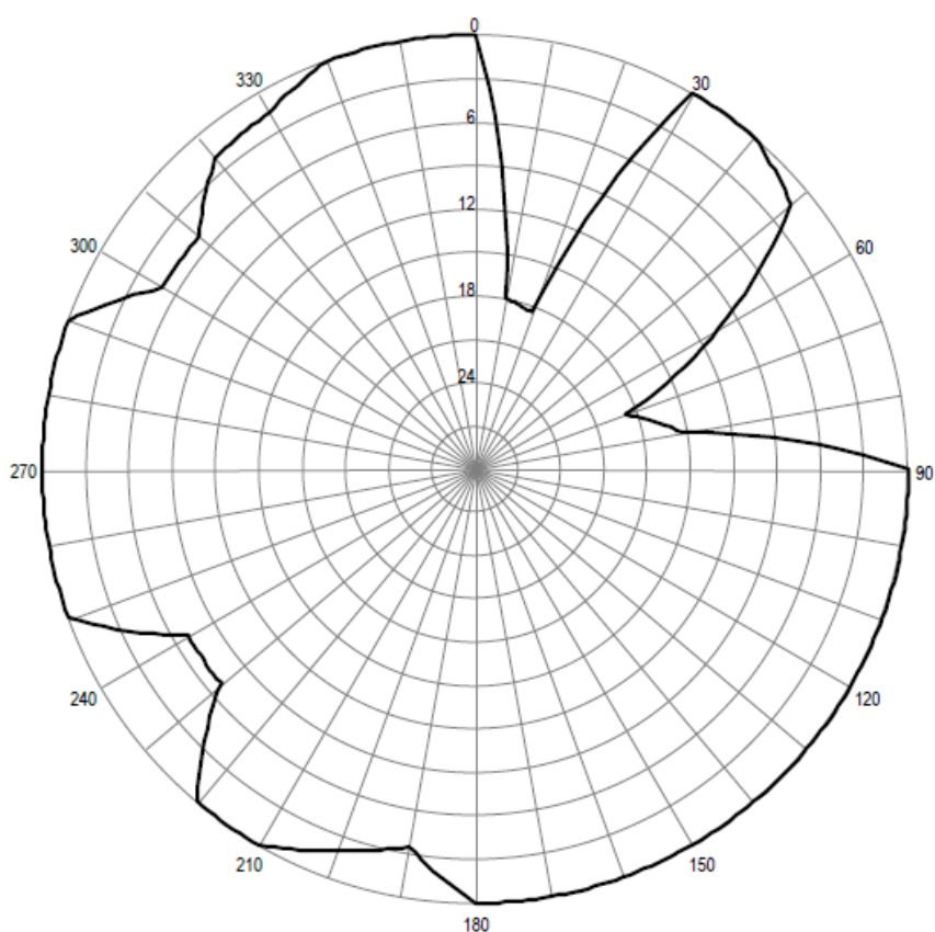
Pozioma charakterystyka promieniowania anteny stacji Porażyn 100,40 MHz
