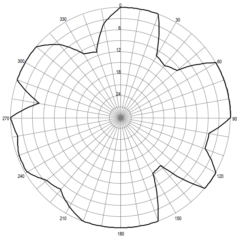
Pozioma charakterystyka promieniowania anteny stacji Babia Góra 97,90 MHz
