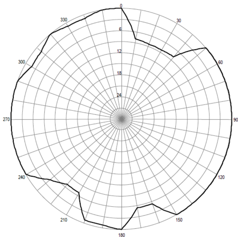
Pozioma charakterystyka promieniowania anteny stacji Augustów 97,70 MHz
