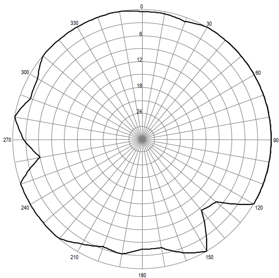
Pozioma charakterystyka promieniowania anteny stacji Białystok 89,20 MHz
