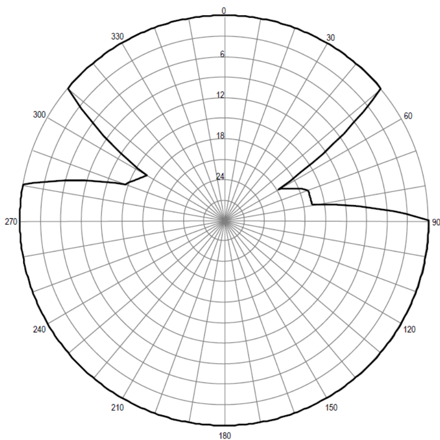
Pozioma charakterystyka promieniowania anteny stacji Słupsk 93,10 MHz
