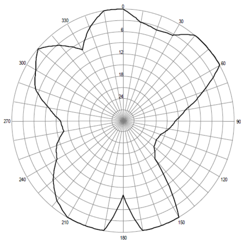
Pozioma charakterystyka promieniowania anteny stacji Kazimierz Dolny 97,20 MHz
