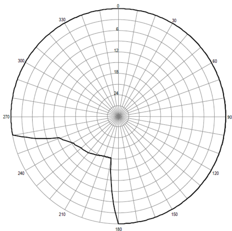
Pozioma charakterystyka promieniowania anteny stacji Lublin 92,90 MHz
