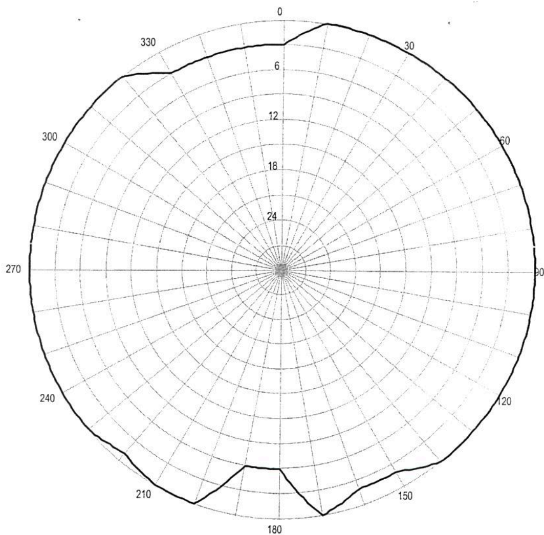
Pozioma charakterystyka promieniowania anteny stacji Zabrze 106,4 MHz
