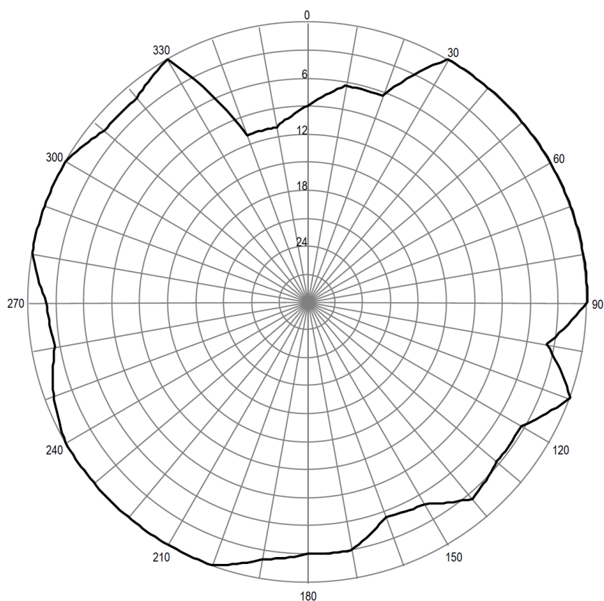
Pozioma charakterystyka promieniowania anteny stacji Konin Brzezińskie Holendry 106,0 MHz
