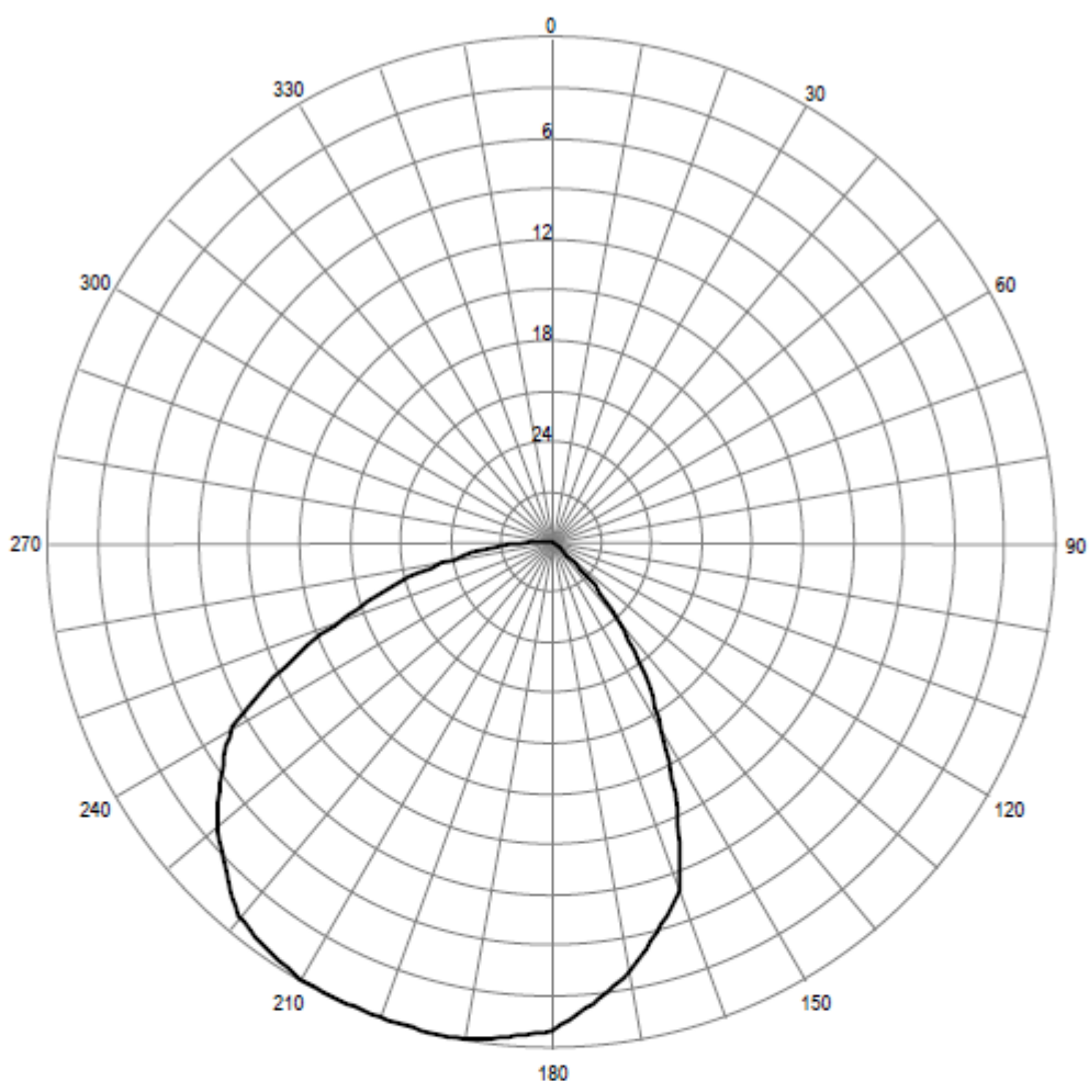
Pozioma charakterystyka promieniowania anteny stacji Łysa Góra Dziwiszów 100,4 MHz
