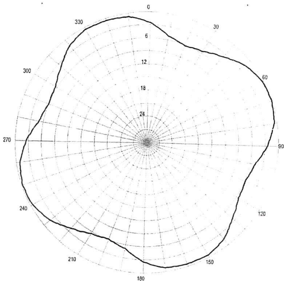
Pozioma charakterystyka promieniowania systemu antenowego (anteny) stacji Warszawa PKiN 107,5 MHz
