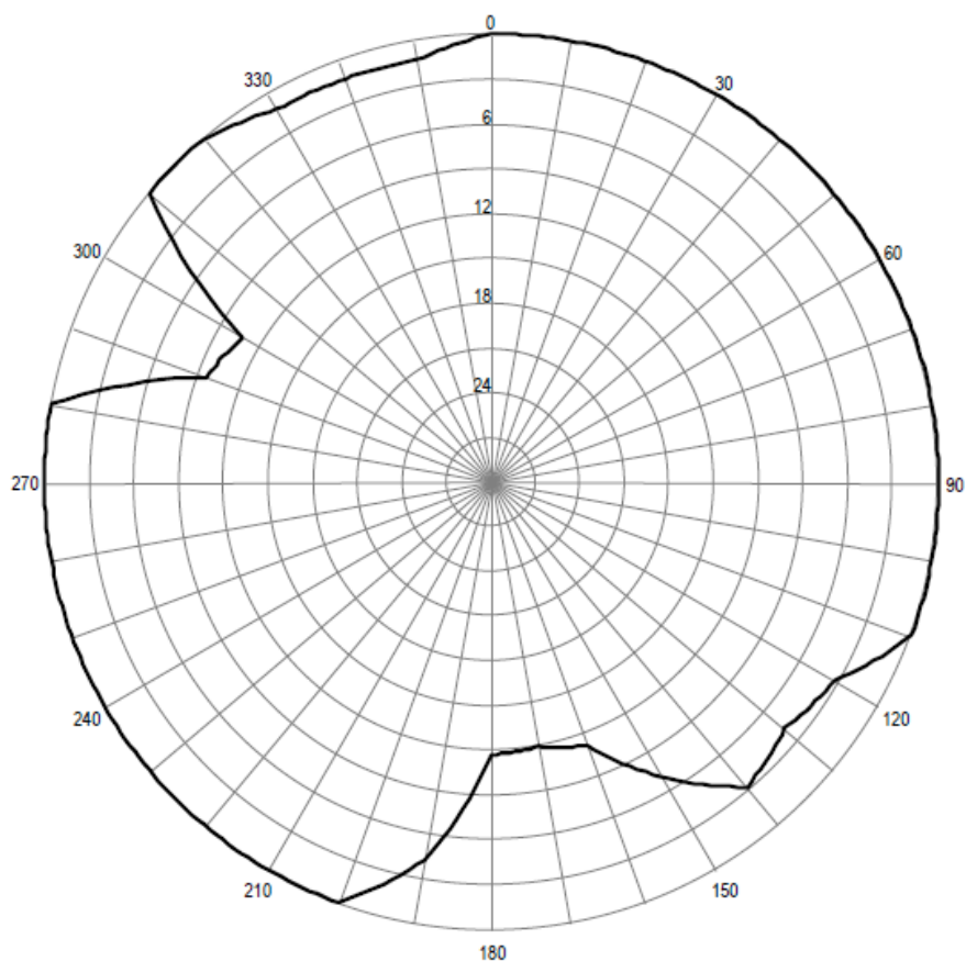
Pozioma charakterystyka promieniowania anteny stacji Puławy 105,80 MHz
