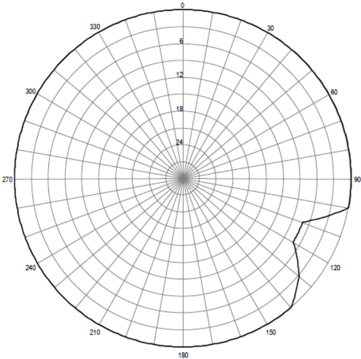
Pozioma charakterystyka promieniowania anteny stacji Słupsk 87,60 MHz
