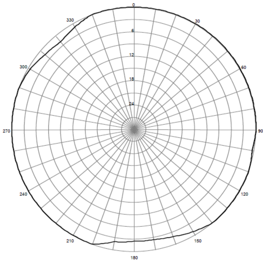
Pozioma charakterystyka promieniowania anteny stacji Kraków 100,50 MHz
