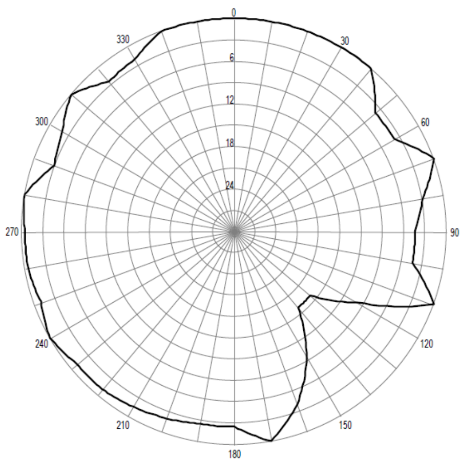
Pozioma charakterystyka promieniowania anteny stacji Kraków 93,70 MHz
