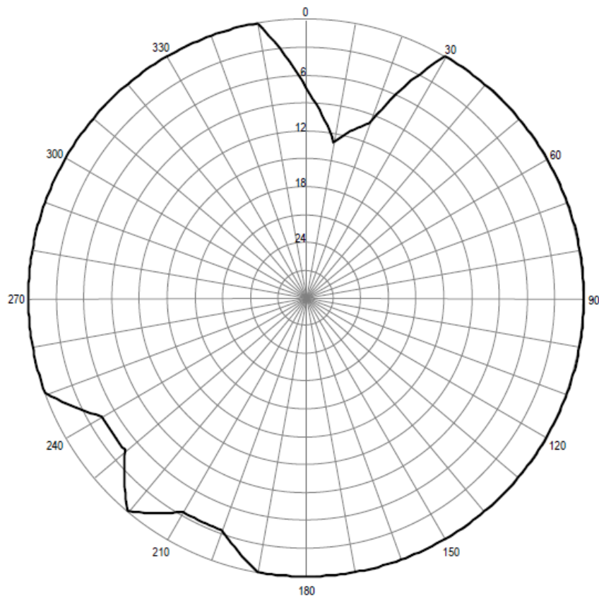
Pozioma charakterystyka promieniowania anteny stacji Białystok 94,80 MHz
