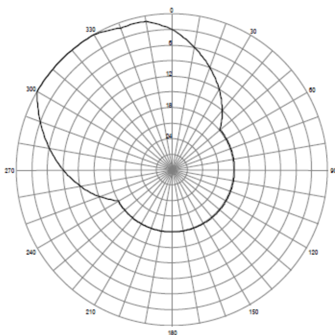
Pozioma charakterystyka promieniowania anteny stacji
