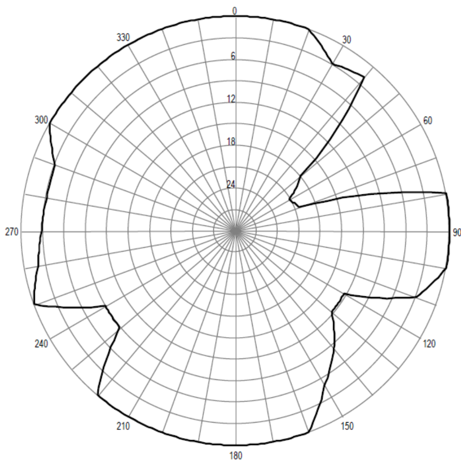
Pozioma charakterystyka promieniowania anteny stacji Chojnice 100,70 MHz
