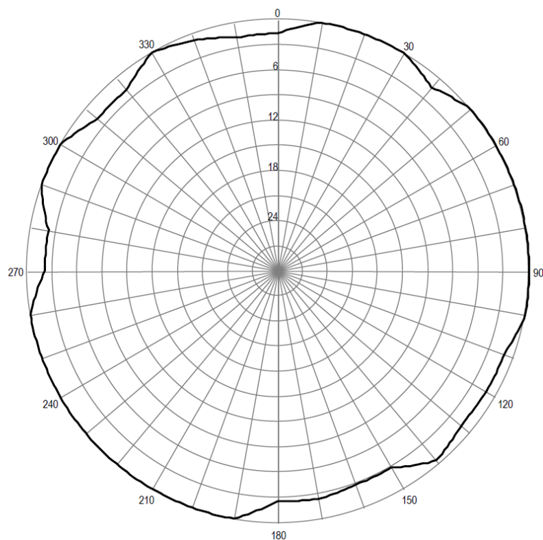
Pozioma charakterystyka promieniowania anteny stacji Suwałki 91,20 MHz
