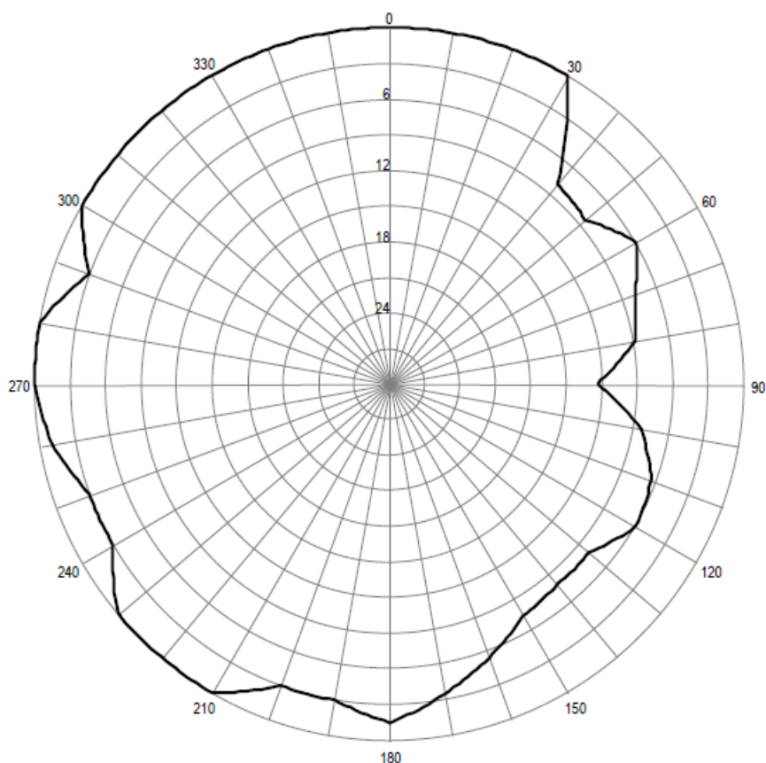
Pozioma charakterystyka promieniowania anteny stacji Gdańsk 104,40 MHz
