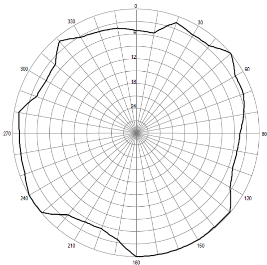
Pozioma charakterystyka promieniowania anteny stacji Warszawa Varso 105,60 MHz
