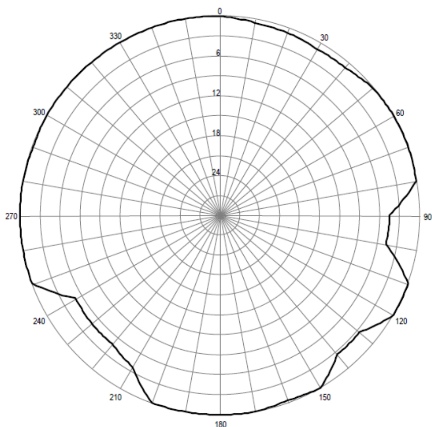
Pozioma charakterystyka promieniowania anteny stacji Warszawa 98,30 MHz
