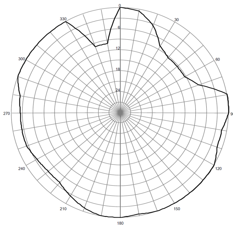
Pozioma charakterystyka promieniowania anteny stacji
