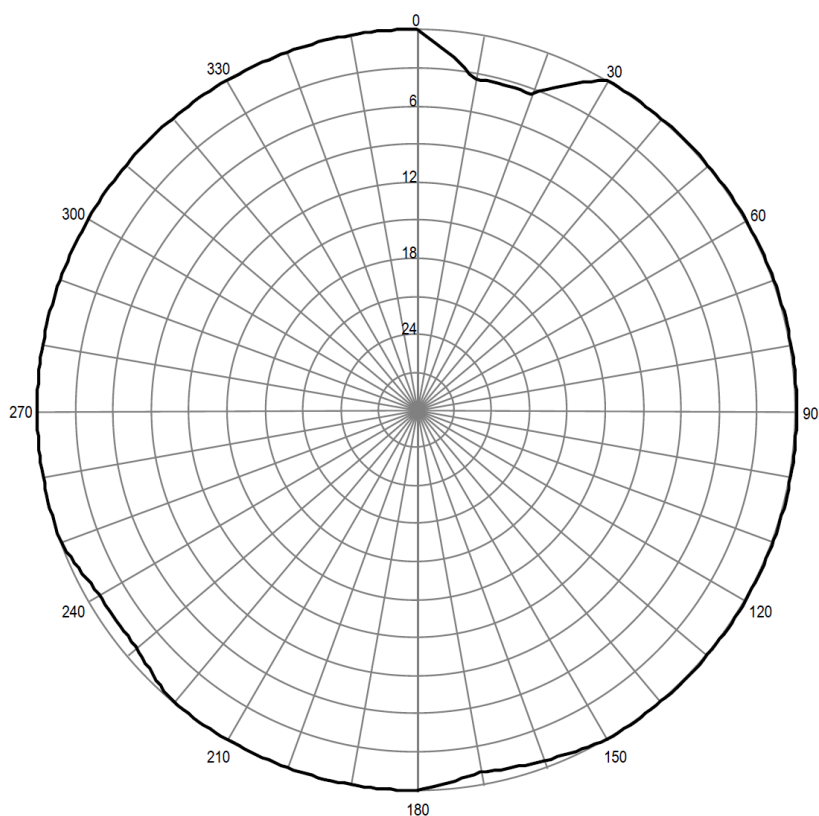
Pozioma charakterystyka promieniowania anteny stacji Ostróda 105,20 MHz
