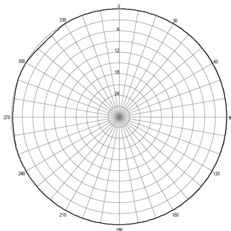
Pozioma charakterystyka promieniowania anteny stacji Bydgoszcz 102,60 MHz
