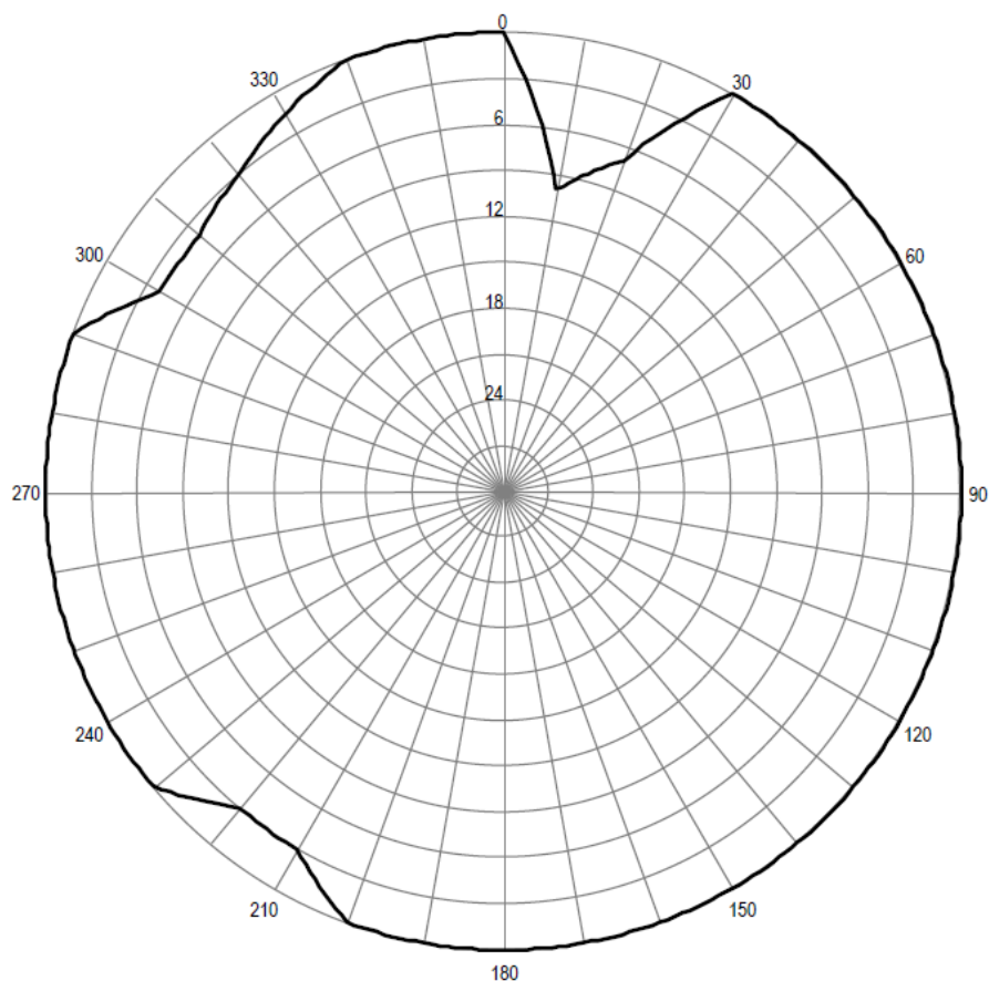
Pozioma charakterystyka promieniowania anteny stacji Gródek 97,20 MHz
