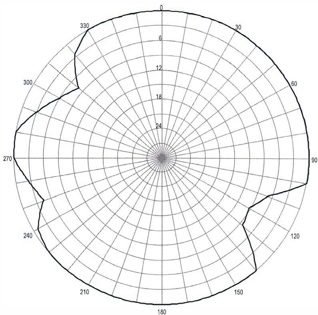
Pozioma charakterystyka promieniowania anteny stacji Opole 99,10 MHz
