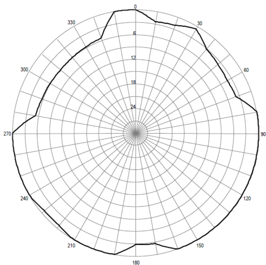
Pozioma charakterystyka promieniowania anteny stacji Warszawa Varso 102,0 MHz
