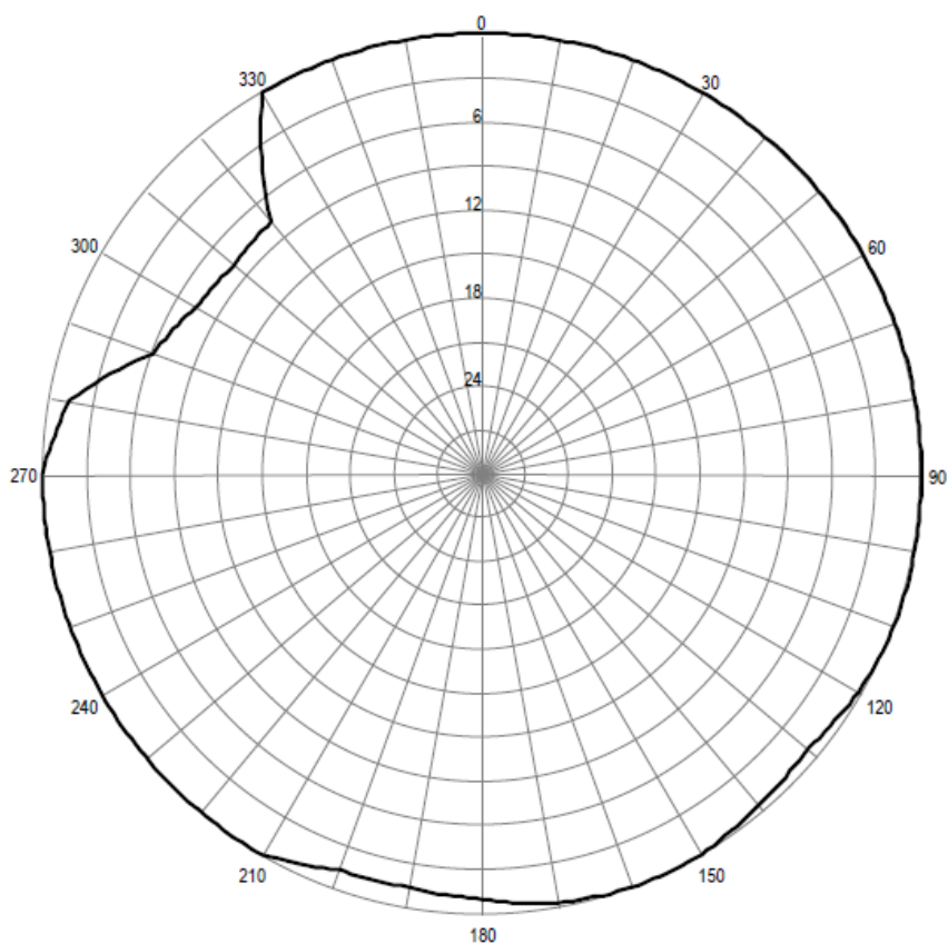
Pozioma charakterystyka promieniowania anteny stacji Sierpc 107,90 MHz
