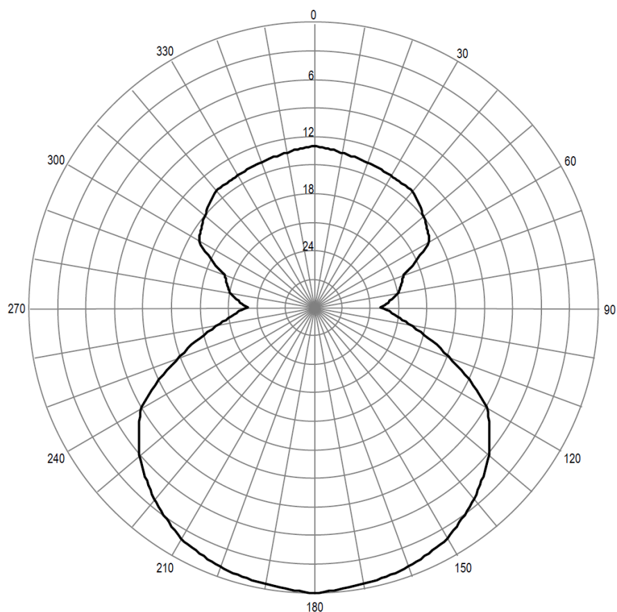
Pozioma charakterystyka promieniowania anteny stacji Wejherowo 102,60 MHz
