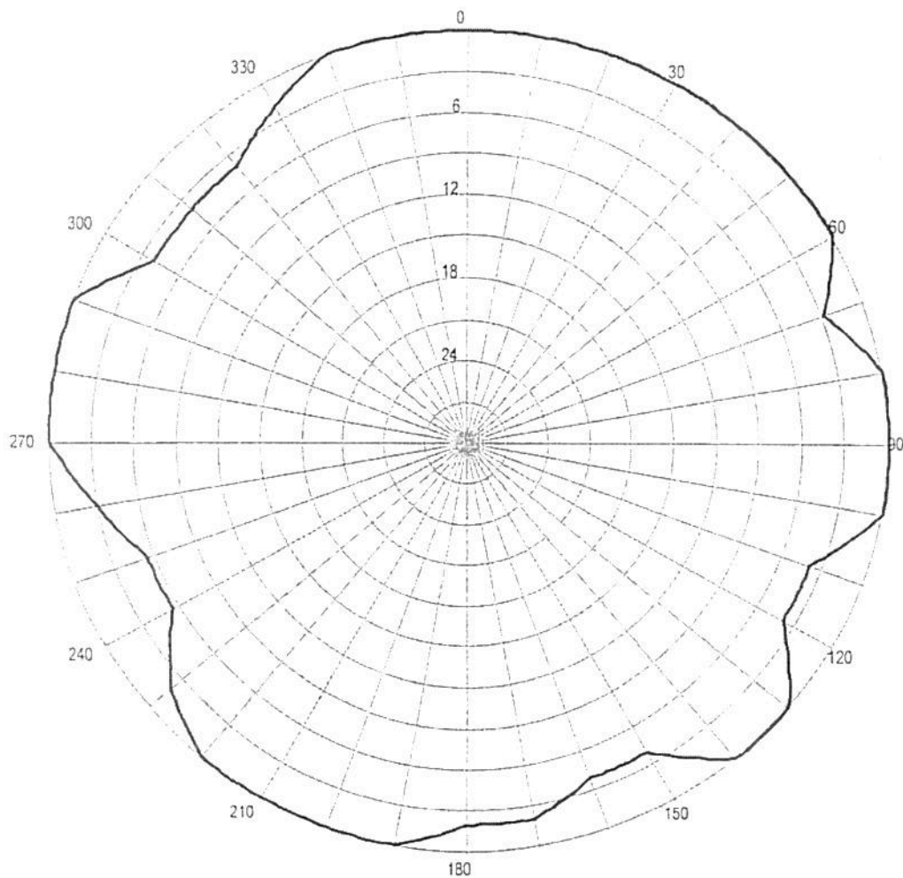
Pozioma charakterystyka promieniowania anteny stacji Opole 97,5 MHz
