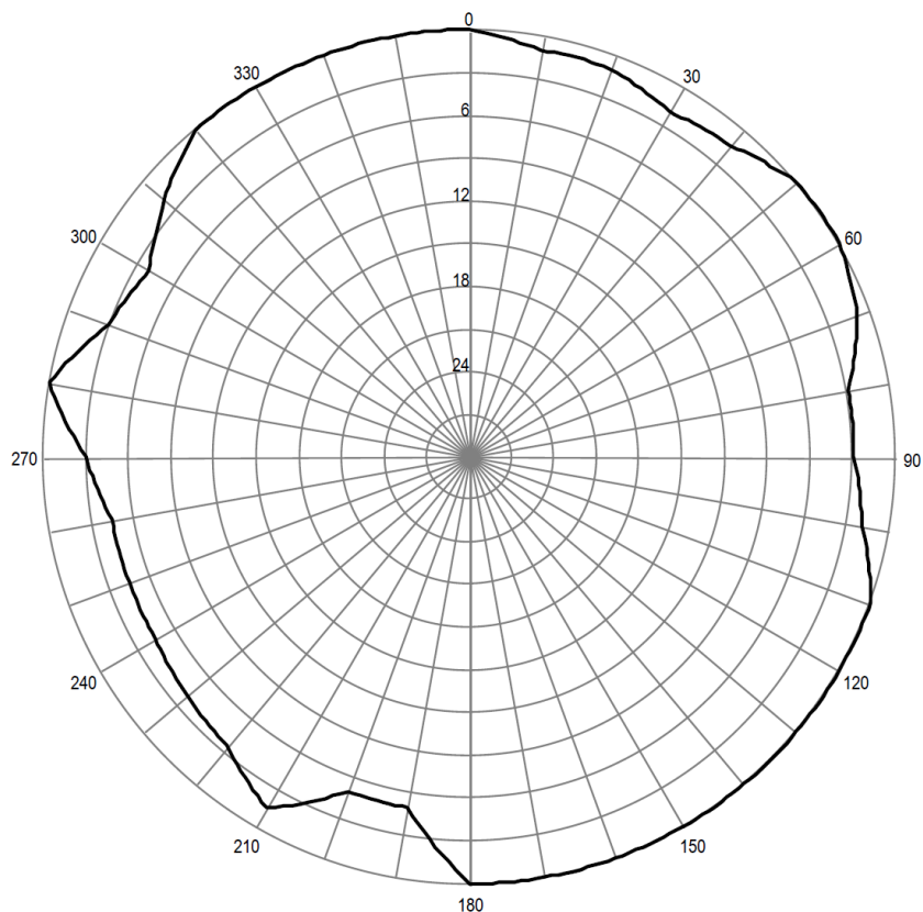
Pozioma charakterystyka promieniowania anteny stacji Będzin 89,80 MHz
