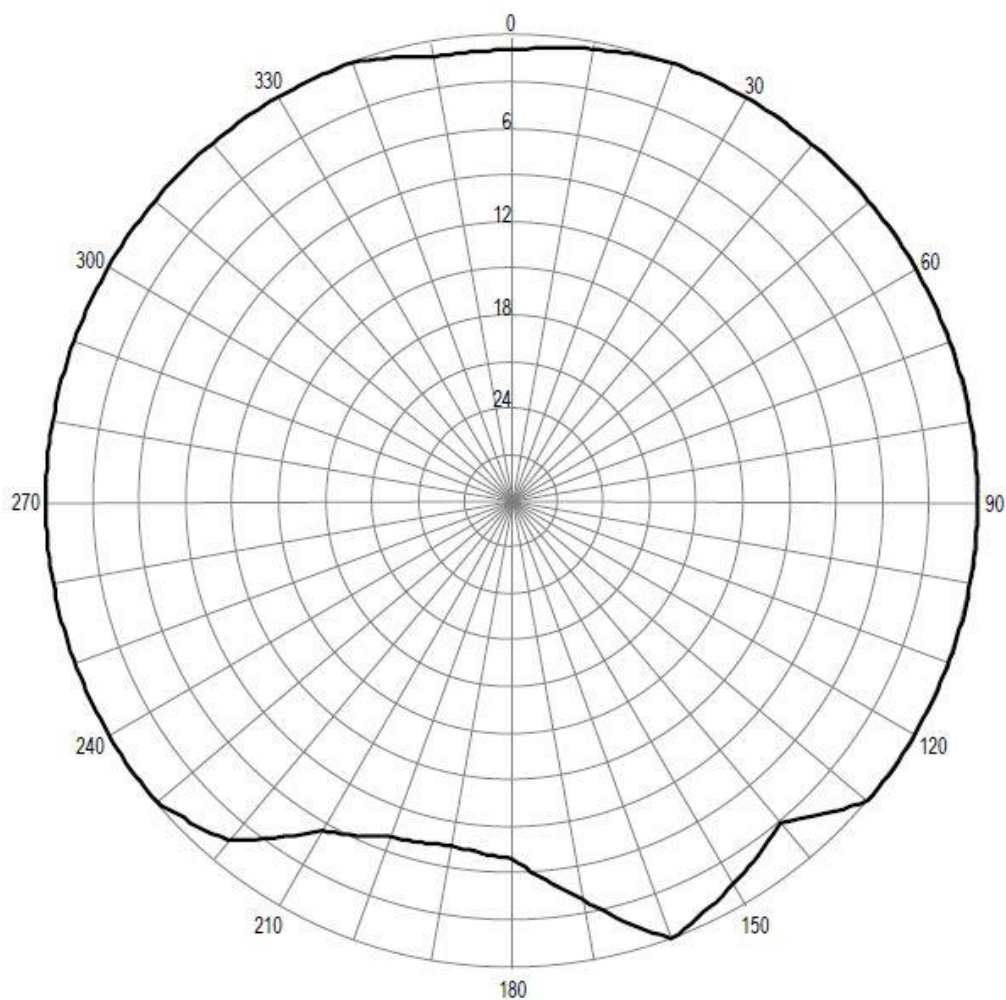
Pozioma charakterystyka promieniowania anteny stacji Stalowa Wola 105,0 MHz
