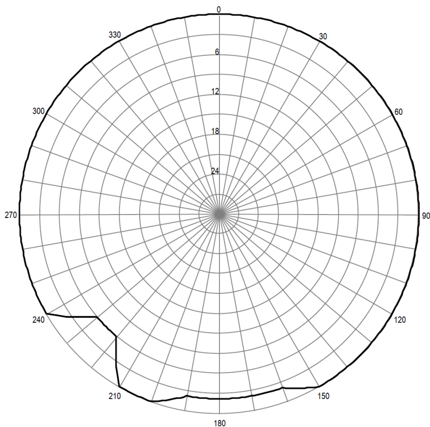
Pozioma charakterystyka promieniowania anteny stacji Namysłów 92,40 MHz
