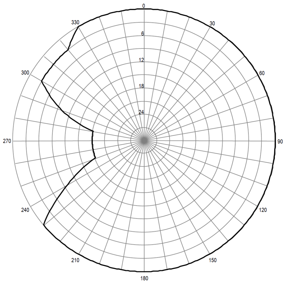
Pozioma charakterystyka promieniowania anteny stacji Nowa Ruda 100,40 MHz
