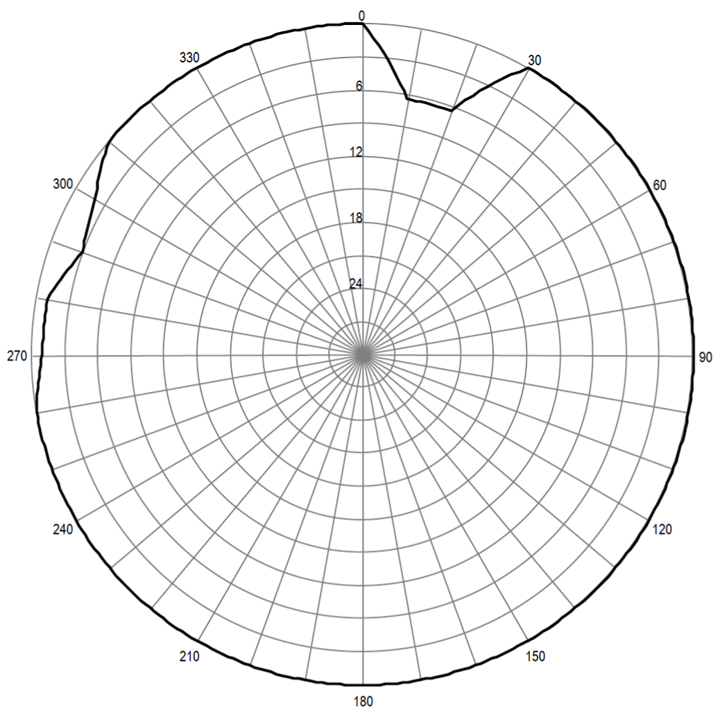
Pozioma charakterystyka promieniowania anteny stacji Stara Góra 90,70 MHz
