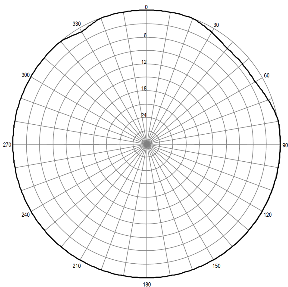
Pozioma charakterystyka promieniowania anteny stacji Świdnica 98,10 MHz
