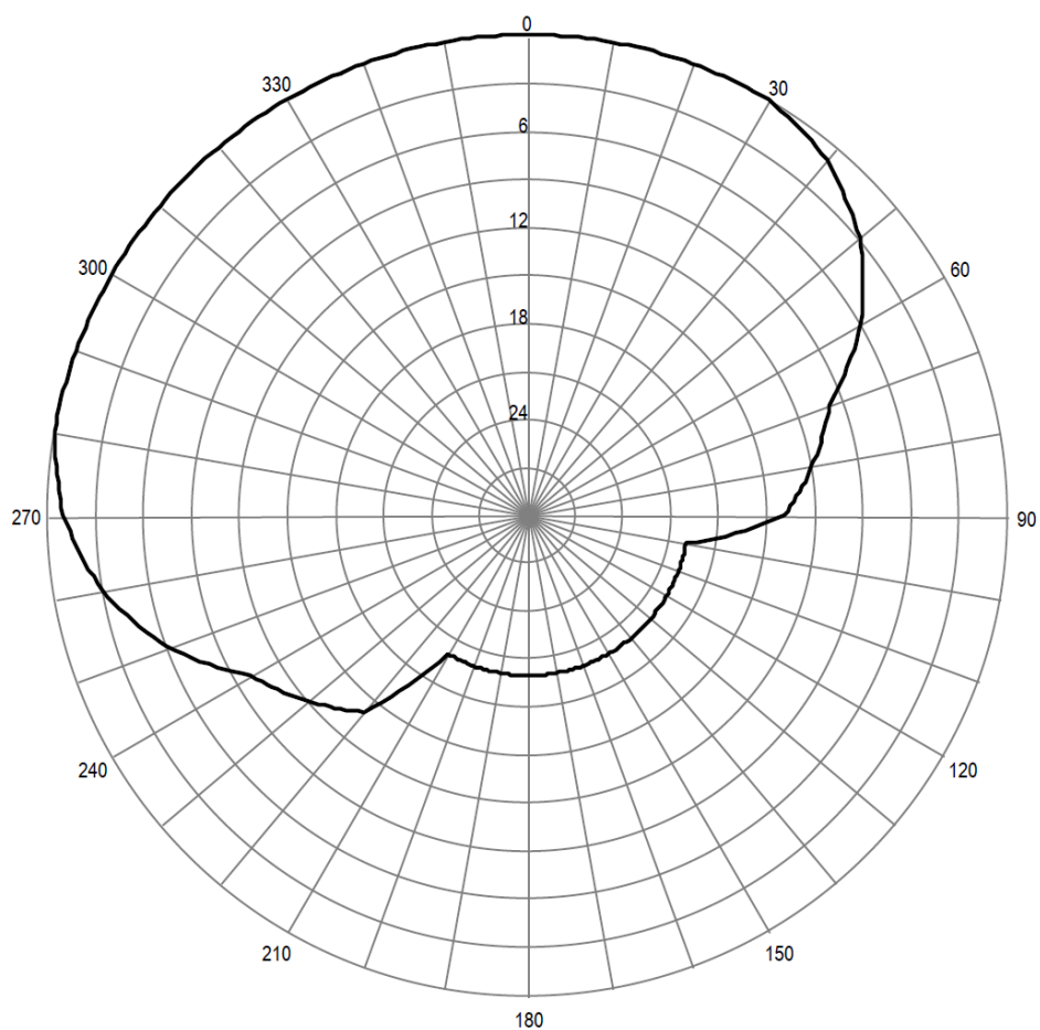
Pozioma charakterystyka promieniowania anteny stacji Bystrzyca Kłodzka 107,20 MHz
