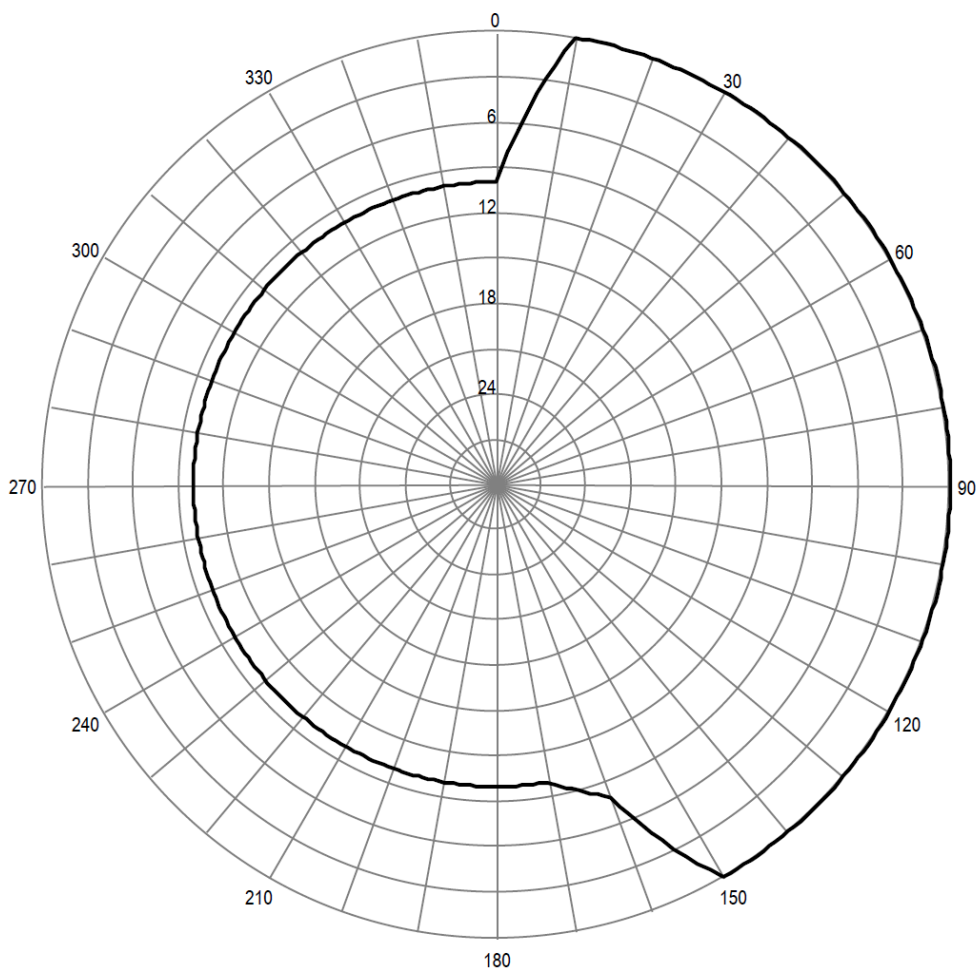
Pozioma charakterystyka promieniowania anteny stacji Jerzykowice Wielkie 88,70 MHz
