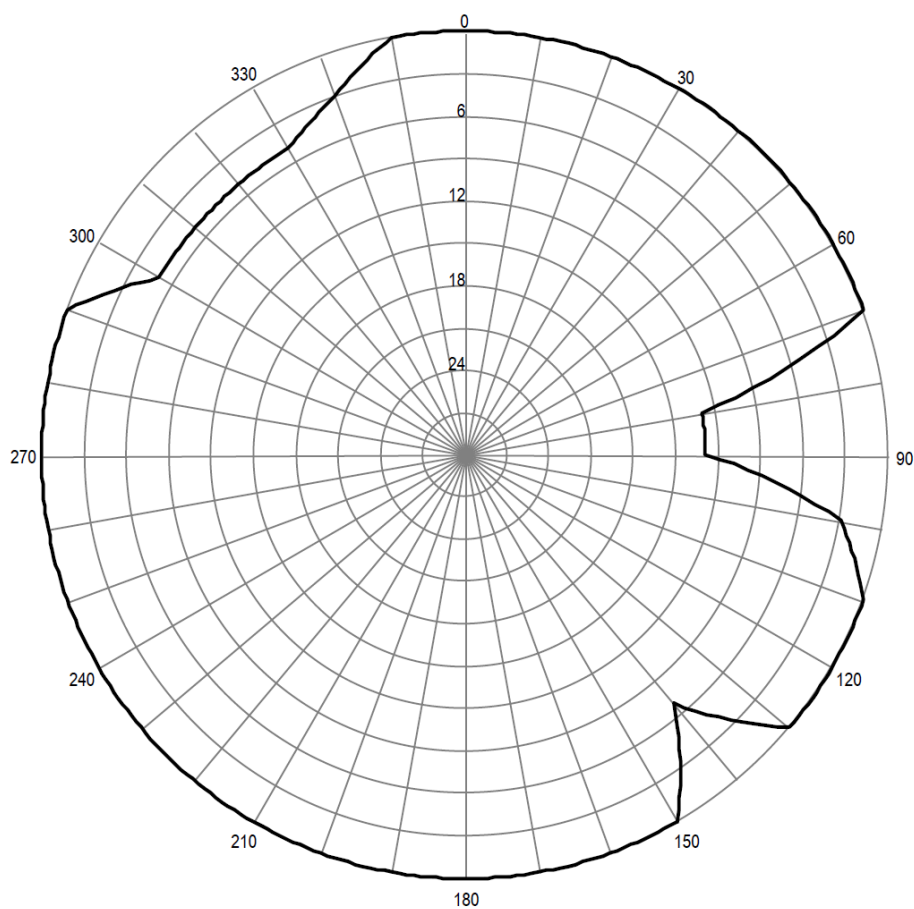
Pozioma charakterystyka promieniowania anteny stacji Strzelin 94,80 MHz
