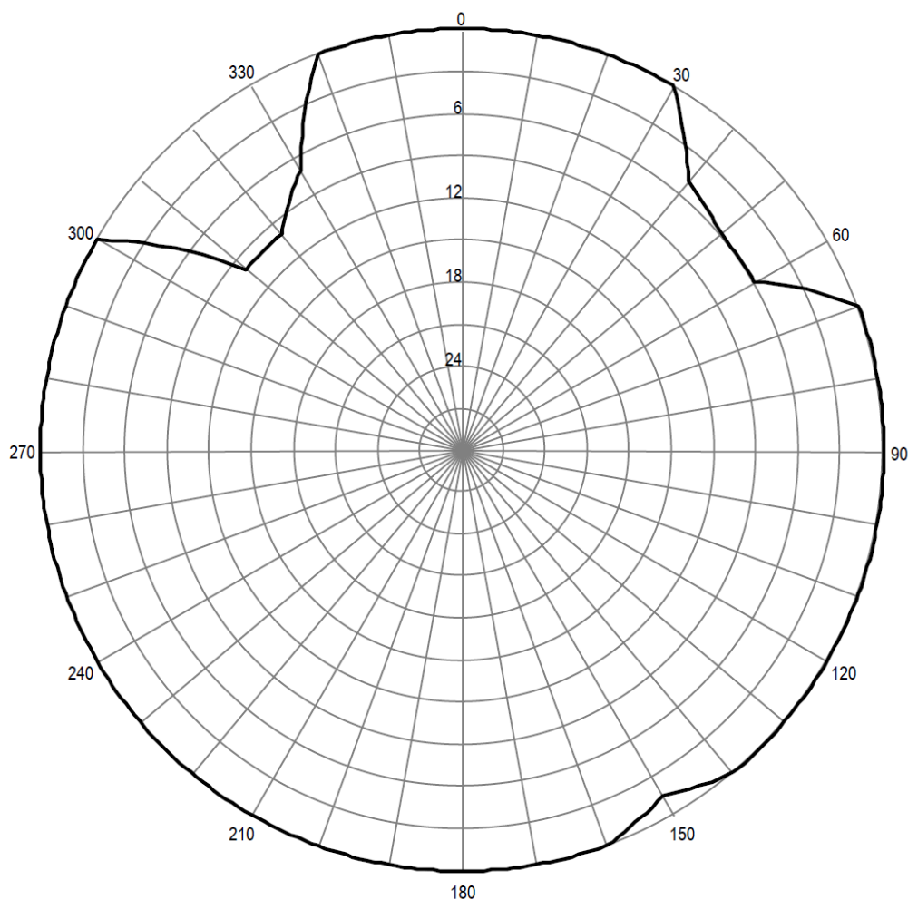
Pozioma charakterystyka promieniowania anteny stacji Kłodzko 97,10 MHz
