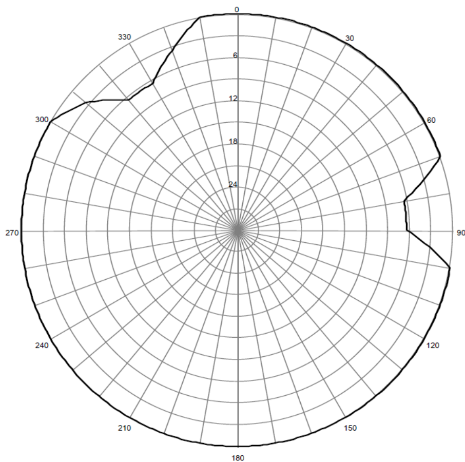
Pozioma charakterystyka promieniowania anteny stacji Kołaczyce 93,30 MHz
