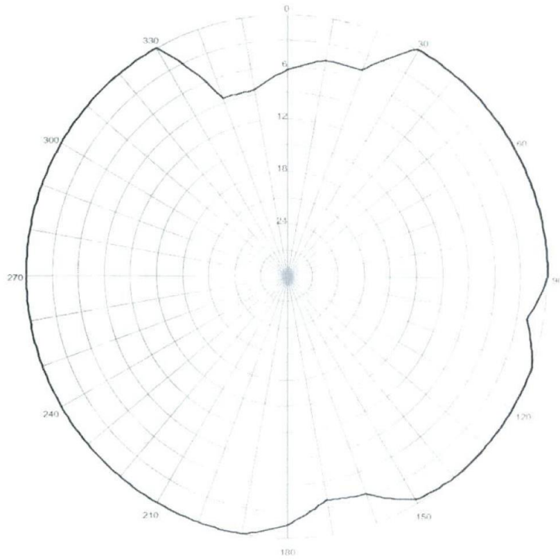
Pozioma charakterystyka promieniowania anteny stacji Paprotnia 106,0 MHz
