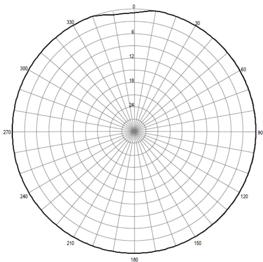
Pozioma charakterystyka promieniowania anteny stacji Dzierżoniów 96,40 MHz
