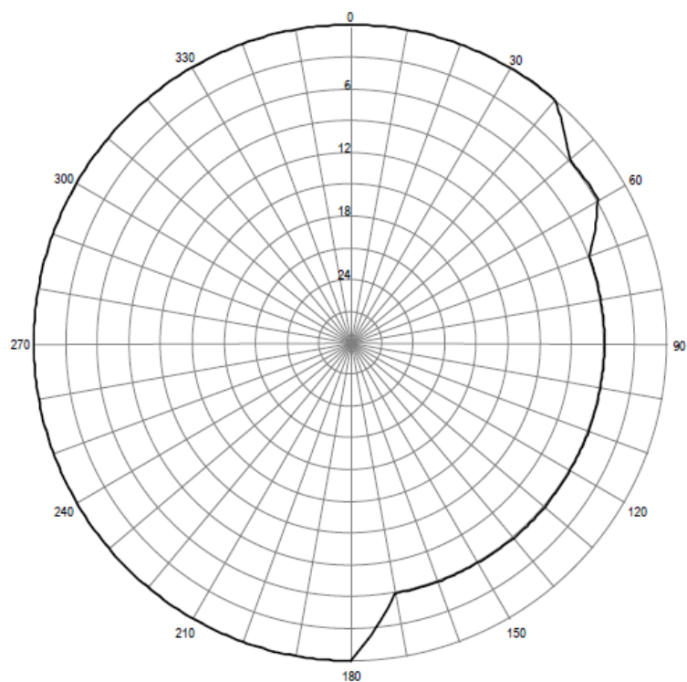
Pozioma charakterystyka promieniowania anteny stacji Tomaszów Mazowiecki 92,90 MHz
