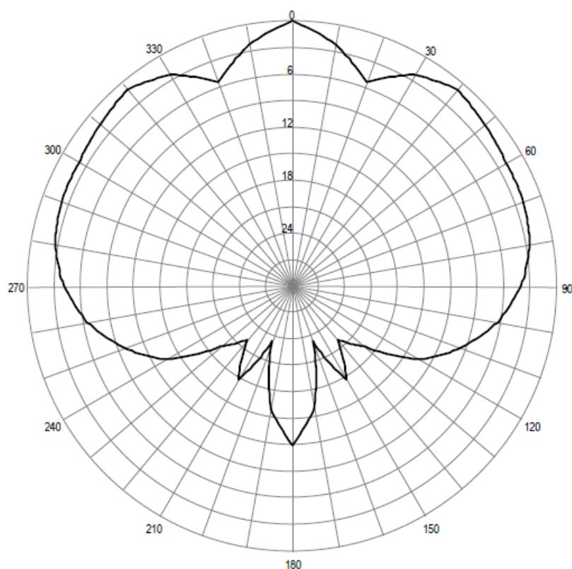
Pozioma charakterystyka promieniowania anteny stacji Krynica G. Parkowa 104,60 MHz
