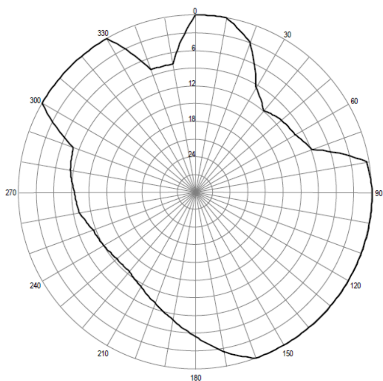
Pozioma charakterystyka promieniowania anteny stacji Gniezno 96,80 MHz
