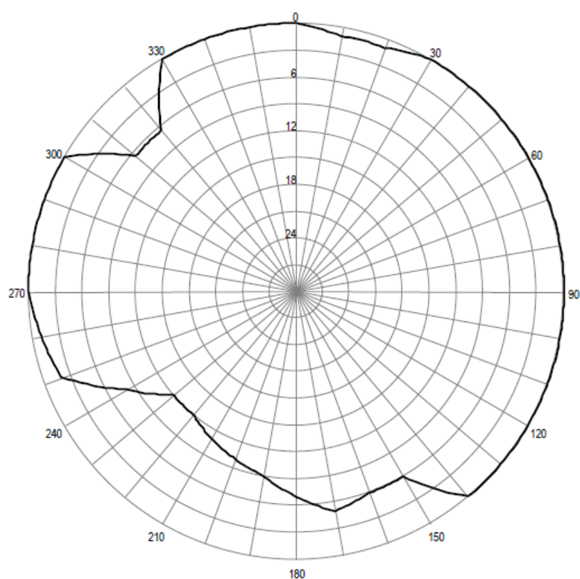
Pozioma charakterystyka promieniowania anteny stacji Wągrowiec 97,20 MHz
