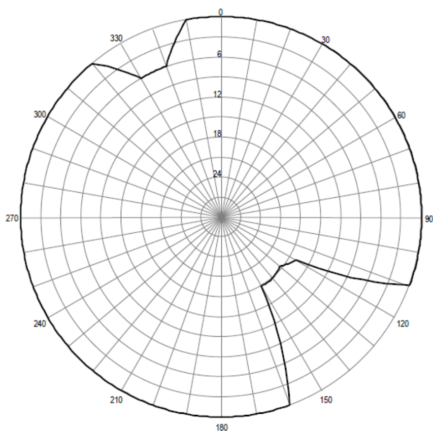
Pozioma charakterystyka promieniowania anteny stacji Janowiec Wielkopolski 99,70 MHz
