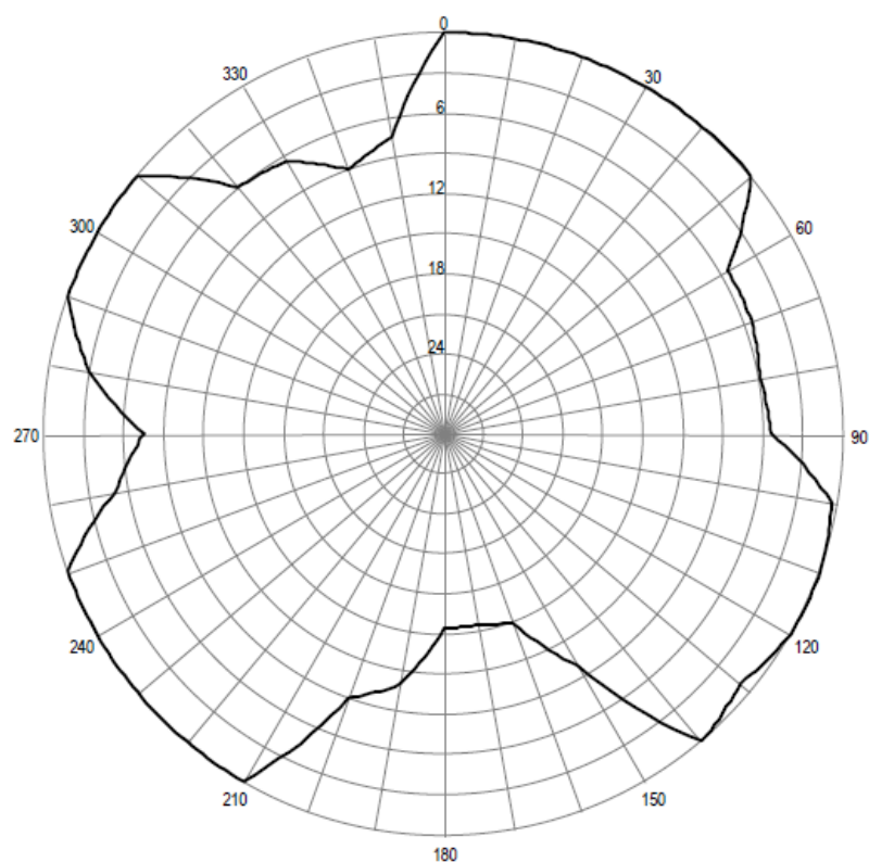
Pozioma charakterystyka promieniowania anteny stacji Piła 107,30 MHz
