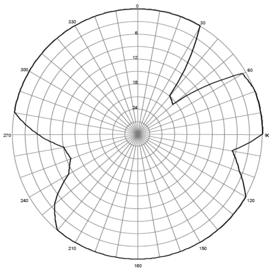
Pozioła charakterystyka promieniowania anteny stacji Mogilno 89,0 MHz
