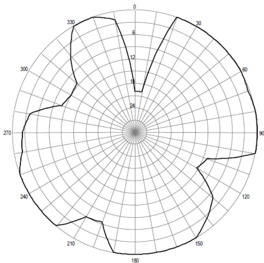
Pozioma charakterystyka promieniowania anteny stacji Gołańcz 105,80 MHz
