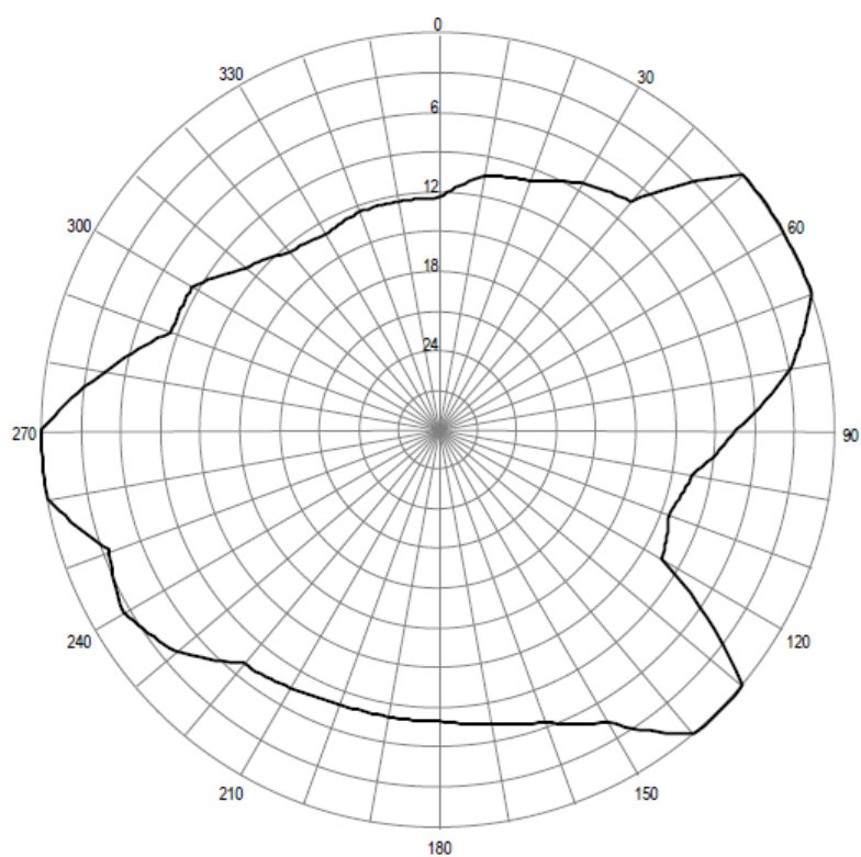
Pozzioma charakterystyka promieniowania anteny stacji Zduńska Wola 92,10 MHz
