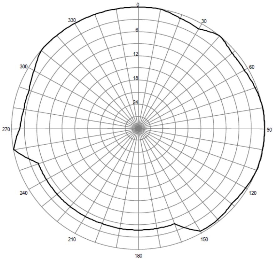
Pozioma charakterystyka promieniowania anteny stacji Wrocław 105,50 MHz
