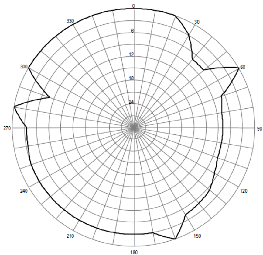
Pozioma charakterystyka promieniowania anteny stacji Nysa 93,10 MHz
