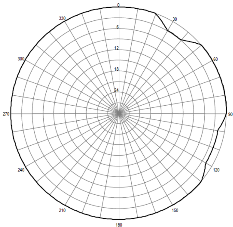
Pozioma charakterystyka promieniowania anteny stacji Tczew 100,80 MHz
