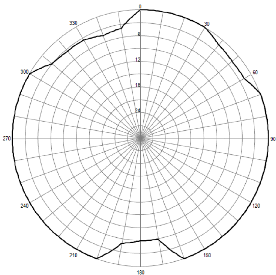
Pozioma charakterystyka promieniowania anteny stacji Ostrzeszów 96,90 MHz
